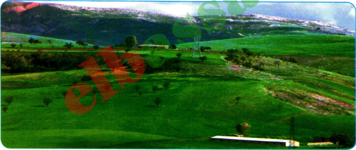
السند 3 : الهضابُ العُليا في الجزائر.
