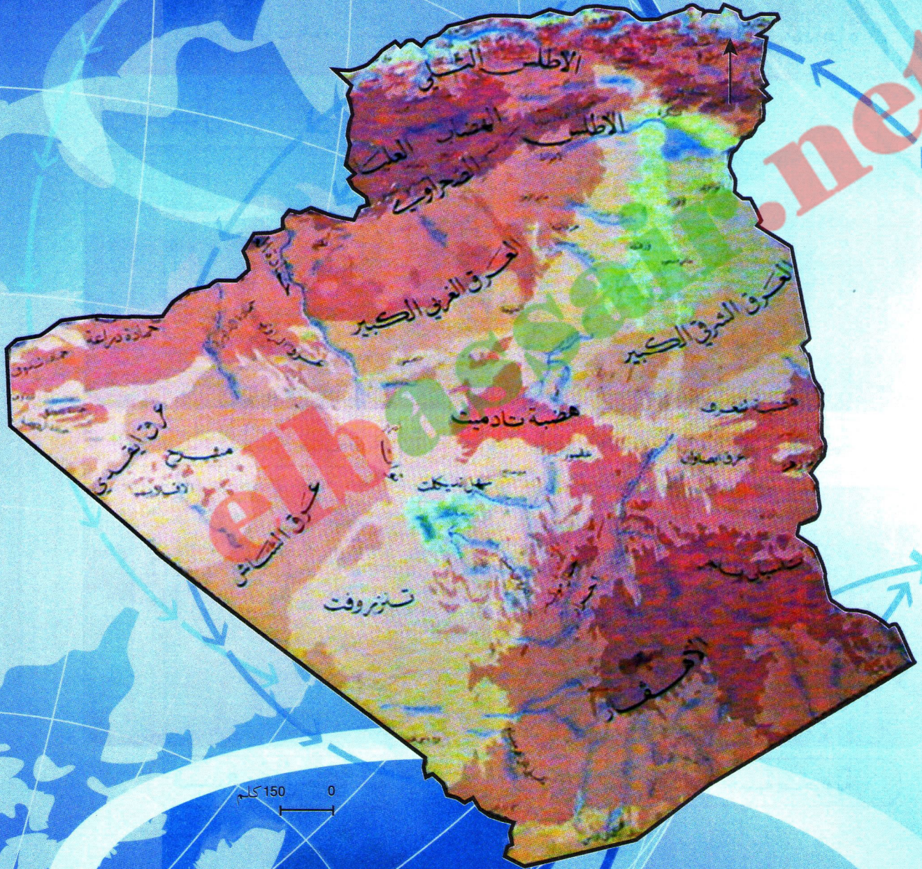
مَظَاهِرُ السَّطْحِ فِي الْجَزَائِرِ
