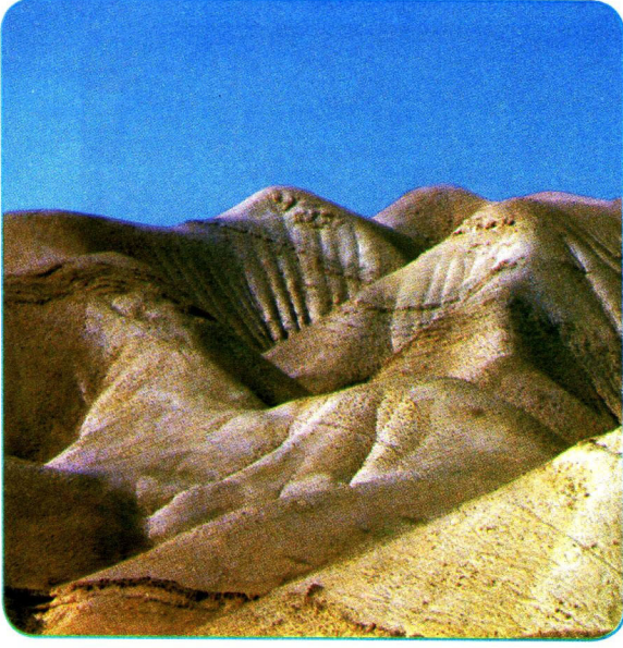
السند : 2 هضابٌ صحراويةٌ.
