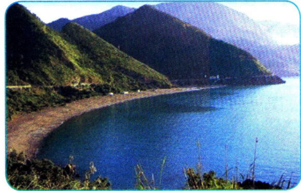
السند 3 : كتل جبليَّة تليَّة
