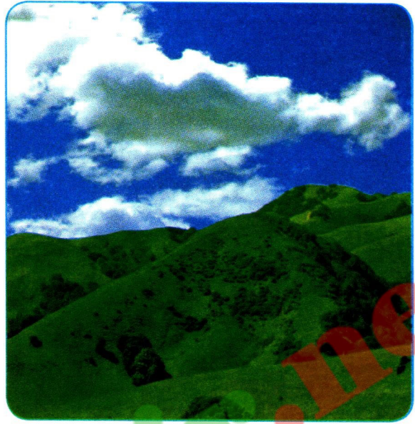
السند : 1 هضابٌ تلمنيةٌ
