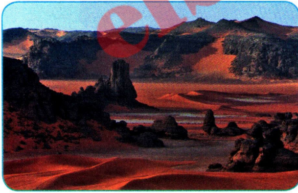
السند 4 : كتل جبليَّة صحراويَّة
